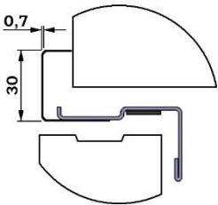
DINTEL REVERSIBLE CON EMBELLECEDOR Reversible lintel with finishing plate / Linteau réversible avec enjoliveur
